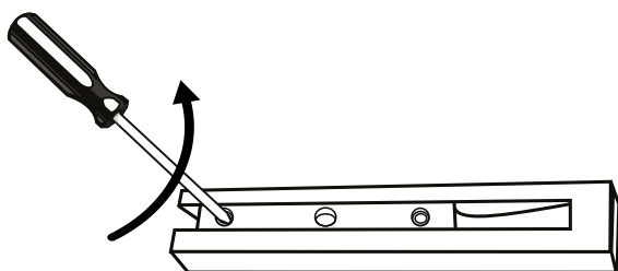
FIGURA 4 Diagrama de cambio de tira de calentamiento.
